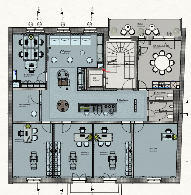
2. Obergeschoss
